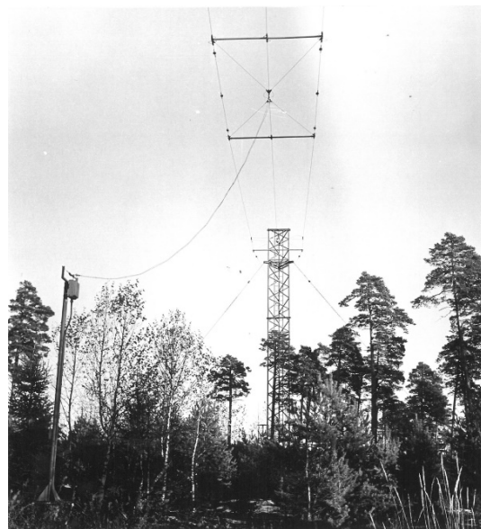
Logperiodisk riktantenn 4 – 30 MHz (vid sändarannex)
