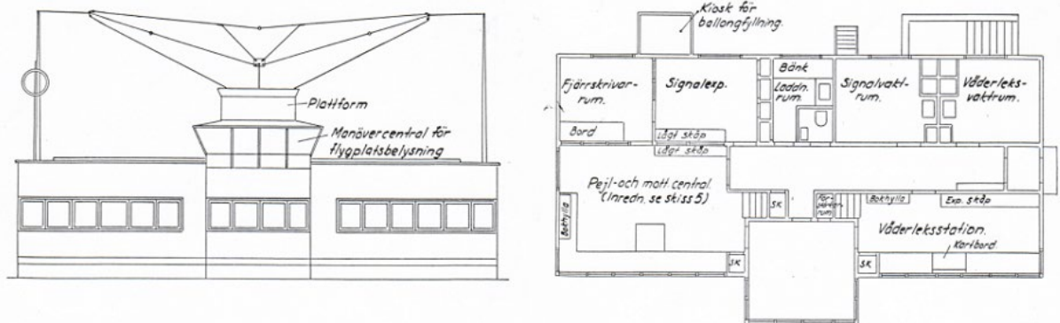
Fast Markradio Typ 1, Installation i kanslihus motsv.
