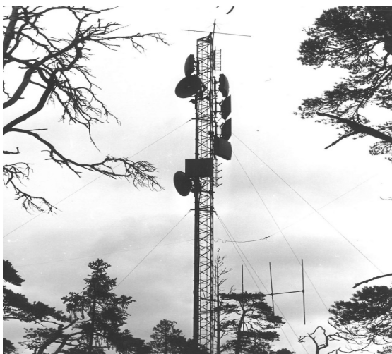
Radiolänkantennerna och 29 MHz Riktantenn mot Us 10
