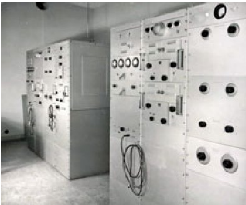
Radiosändare FMR 1 fr v Långvågsdel och Kortvågsdel Sändarnas effektsteg utgjordes av tre Philips PB 3/800 i parallell och gav uteffekten 2,2 kW
