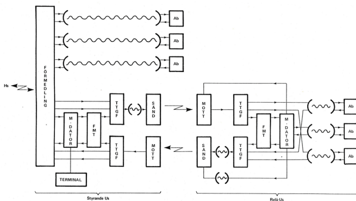
FUNK Principschema
