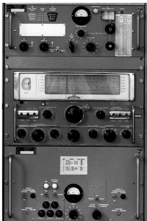
Radiomottagare MRM 8 med Mottagaroscillator 9FE100 och F1-demodulator 9FY100
