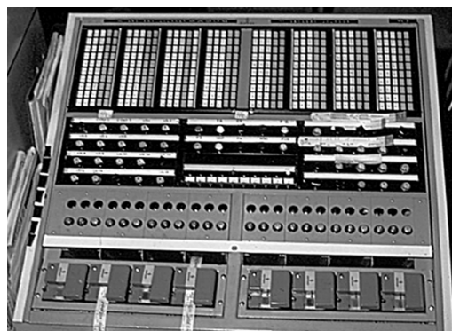
LVA2 Betjäningsbord
