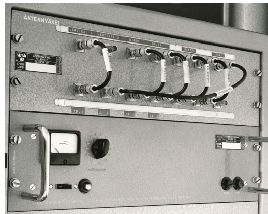
Antennförstärkare NV4 med Antennförväxel
