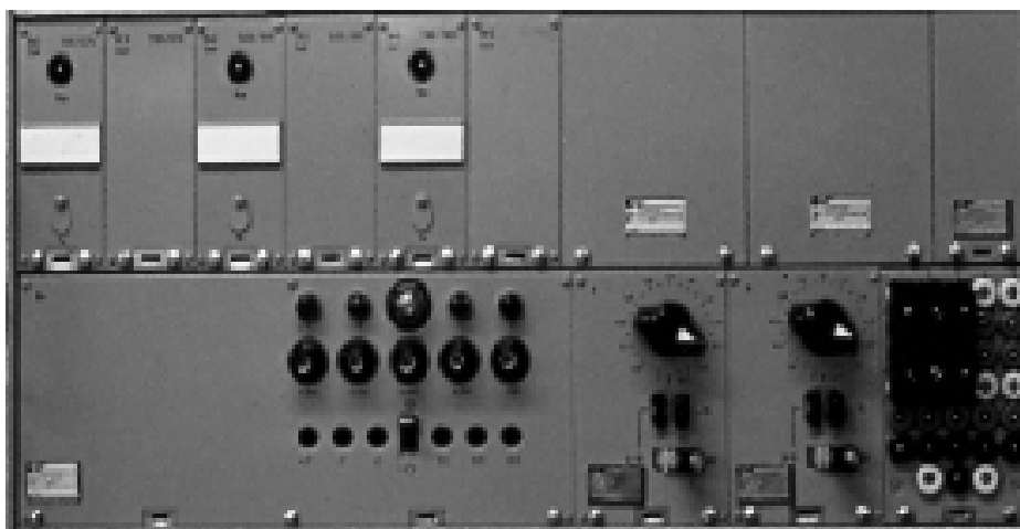
Tontelegrafutrustning WTK340 Sändarram med 3 kanaler
