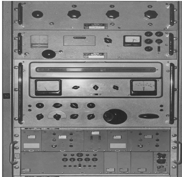
Radiomottagare EK11 med Oscillator NO261 och Demodulator WTK340
